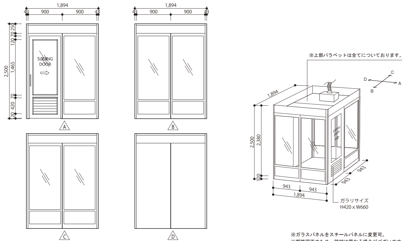
1900 × 1900 4人ユニット正面図
